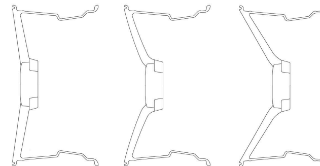
Flaches Profil
